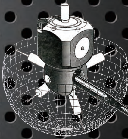
Renishaw Probe & Styli
