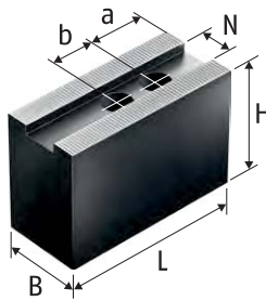
Weiche Aufsatzbacken KM-WB gerade Stahl 16MnCr5 einsatzhärtbar Soft top jaws KM-WB straight Steel 16MnCr5 suitable for case hardening
