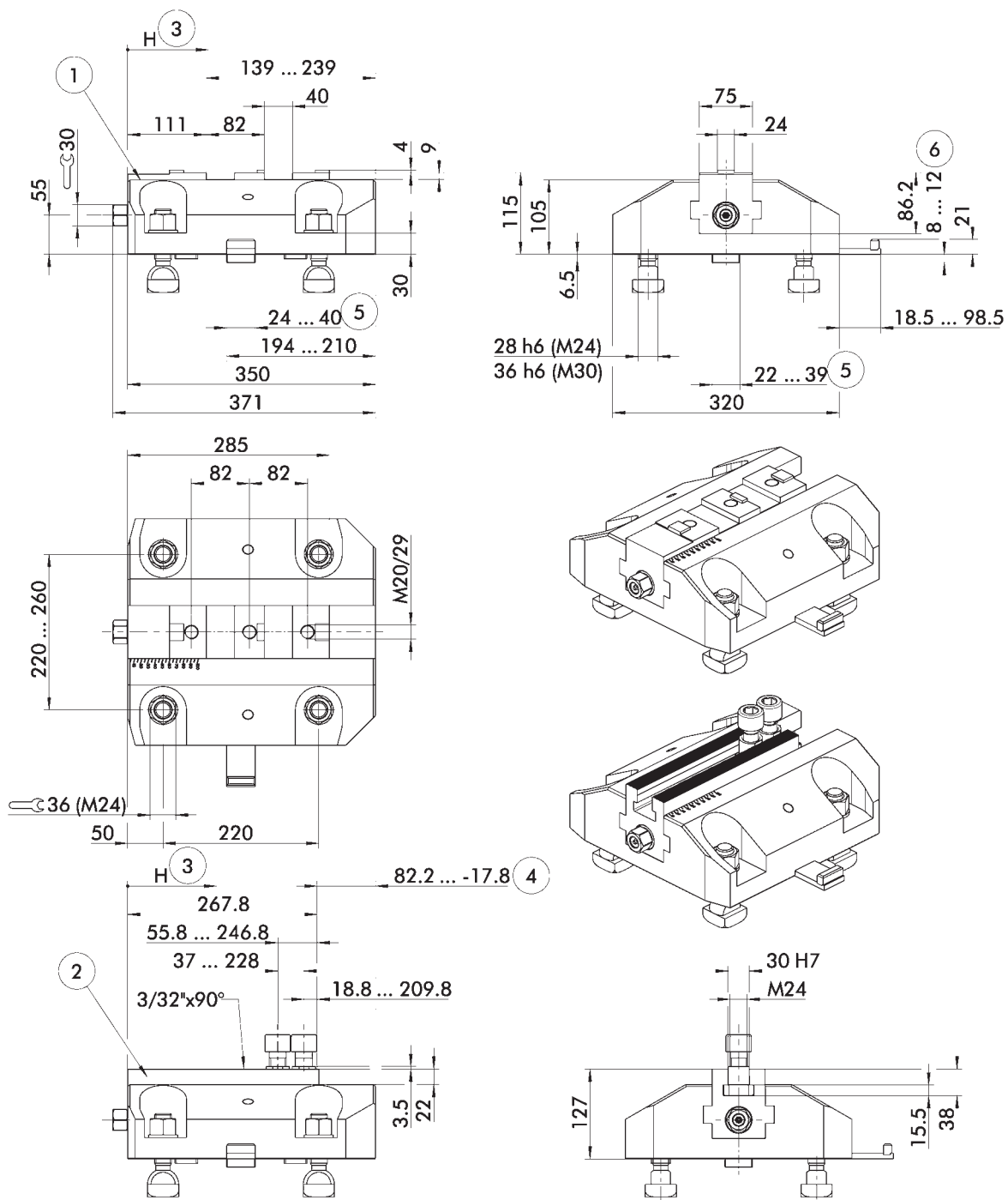
Spannklauenkasten für Aufspannscheiben mit T-Nuten in eingefahrener Stellung dargestellt. Darstellungen inklusive Montagezubehör. Technische Änderungen vorbehalten.
