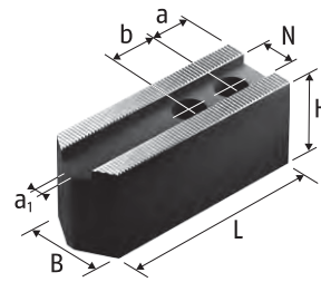
Weiche Aufsatzbacken SWBL Stahl 16MnCr5 einsatzhärtpbar Soft top jaws SWBL Steel 16MnCr5 suitable for case hardening
