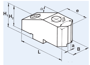
5 Gewichtserleichterung schräg und Anchrägung 60° oder 120°
