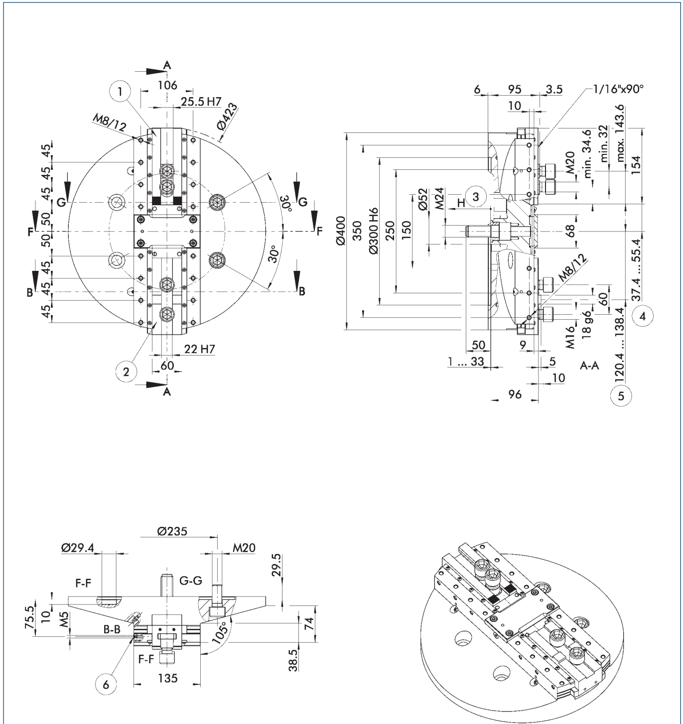
Anschlag nach vorne im Zylinder, nach hinten im Flansch. In der Zeichnung sind zwei Backschnittstellen dargestellt. Technische Änderungen vorbehalten.
