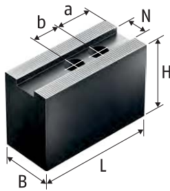
Weiche Aufsatzbacken SWB-FR gerade, SP-WB, SWB, 2 SWK, CWB Stahl 16MnCr5 einsatzhärtpbar Soft top jaws SWB-FR straight, SP-WB, SWB, 2 SWK, CWB Steel 16MnCr5 suitable for case hardening
