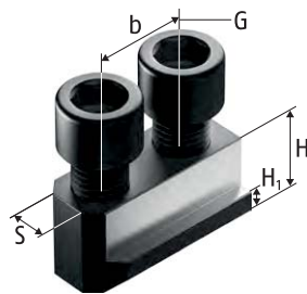
Nutenstein NK T-nut NK
