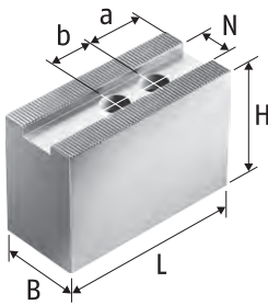
Weiche Aufsatzbacken KM-WBAL Aluminium Soft top jaws KM-WBAL Aluminum
