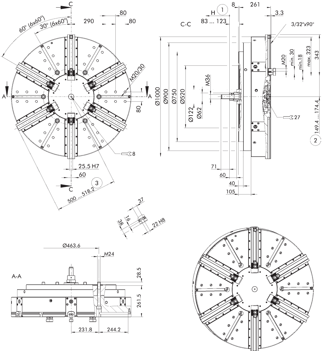
Futter für Wellenspannung in geöffneter Stellung dargestellt. Pendelausgleich in Mittelstellung dargestellt. Technische Änderungen vorbehalten.
