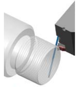
Пример переплетения стружки в клубки
