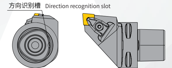
左手刀示例 Example of Left holder
